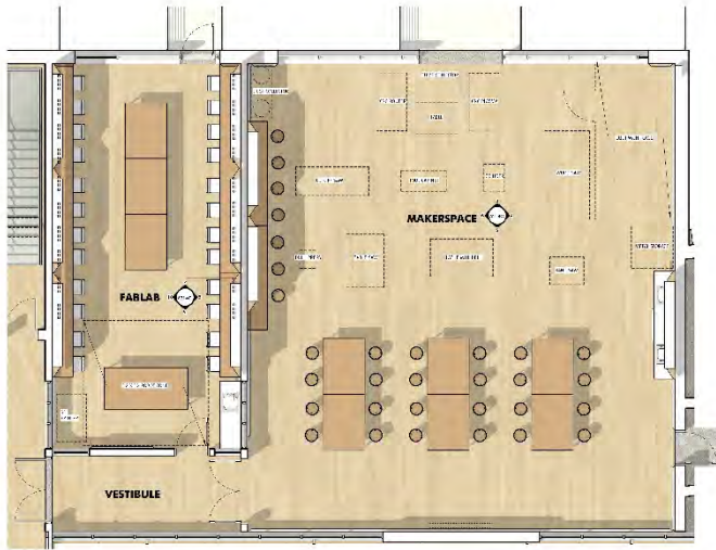
PLAN - FABLAB AND MAKERSPACE
